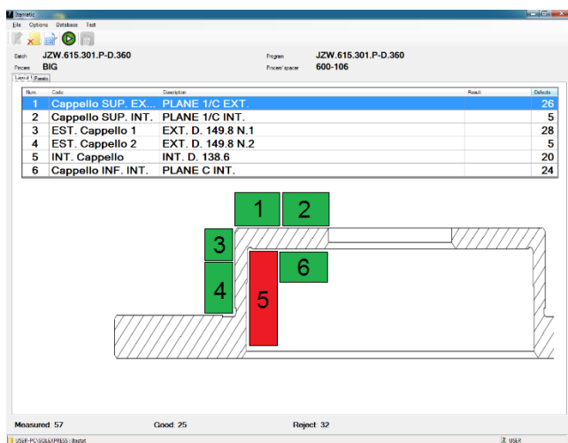
Informazioni relative al pezzo misurato e colonna riassuntiva scarti per singola area controllata
